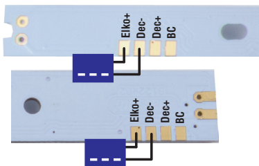
Abbildung 2: Anschluss Pufferelko oder Spannungspuffer Figure 2: Connection power buffer or Power Cap
