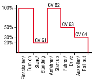
Abbildung 6: Belegung von Takteingang und Taktausgang Illustration #6: Contact Assignment of Clock IN and Clock OUT
