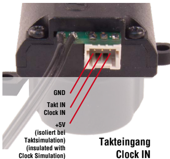
Abbildung 4: Belegung von Takteingang und Taktausgang Illustration #4: Clock Assignment of Clock IN and Clock OUT
