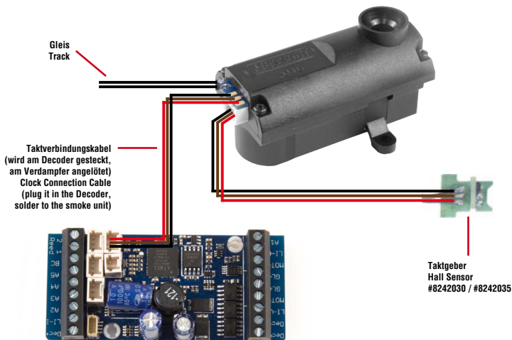
Abbildung 3: Schematische Darstellung des Taktgeberanschlusses Illustration #3: Scematic illustration of the Hall sensor installation
